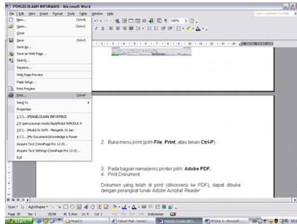
Gambar 23. Menu Print
